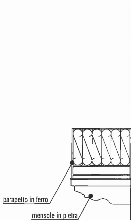
VISTA LATERALE
